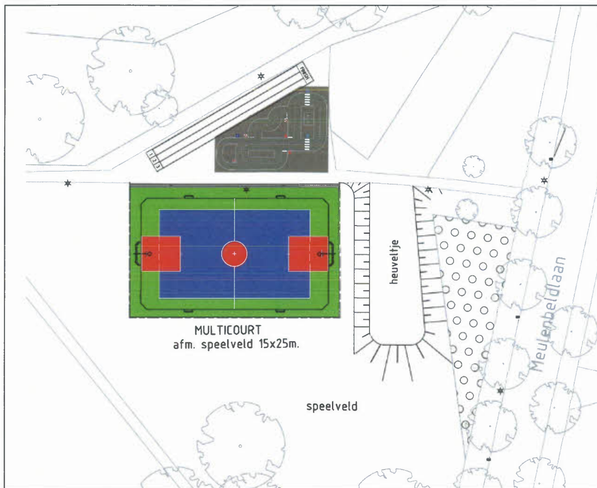
Inrichtingsplan Multicourt Haghoekspark
